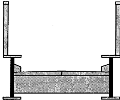
<断面図>
