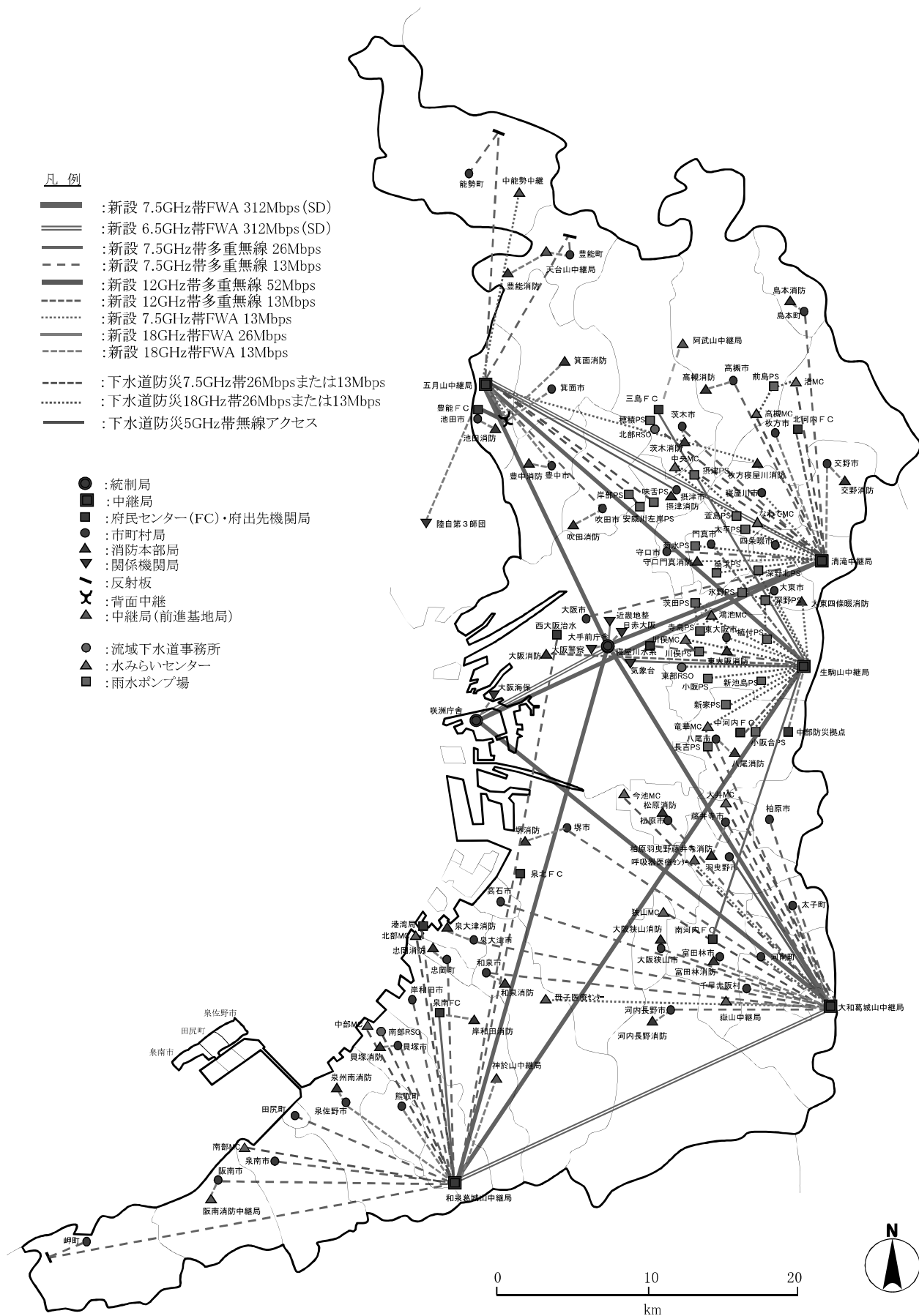
資料1-3:大阪府防災行政無線回線系統図
