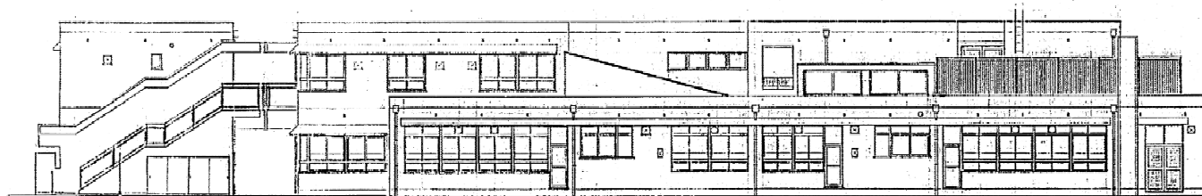
正面図 1/100
