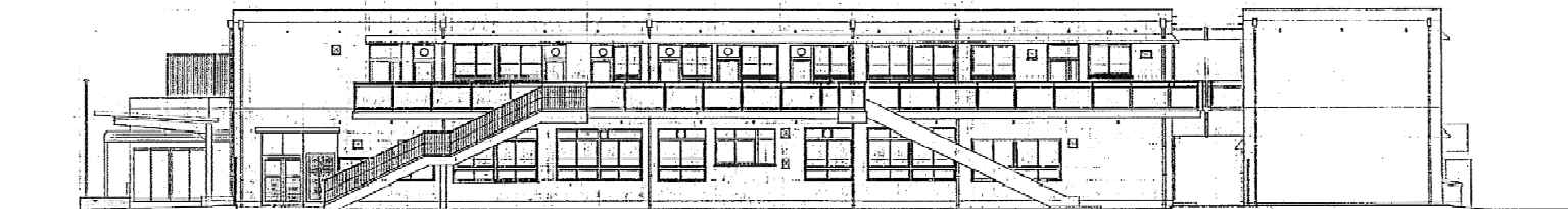
側面図 1/100
