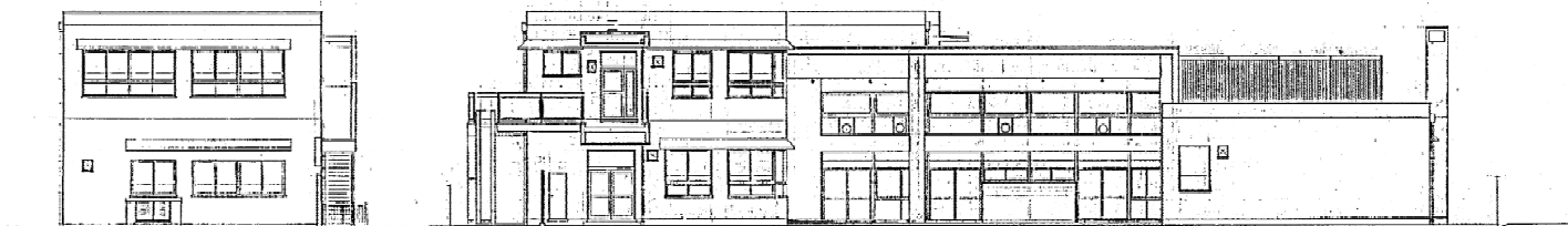
背面図 1/100
